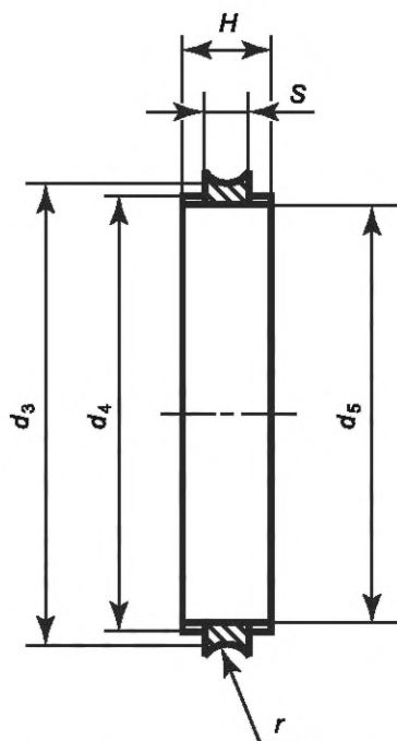
Рисунок 5 — Центрирующее кольцо
