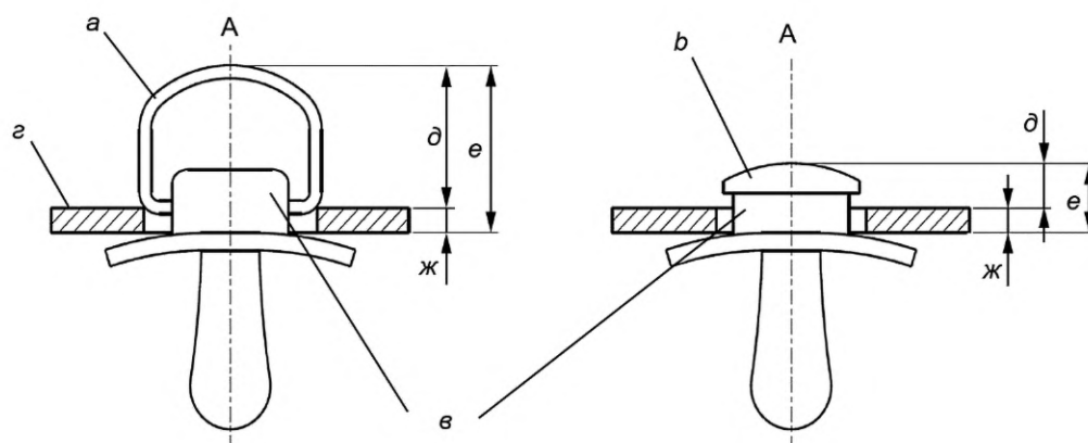
Рисунок 19 — Измерение эффективной глубины проникновения кольца и/или головки, крышки и/или заглушки из гибких материалов с помощью шаблона для испытания защитного диска
