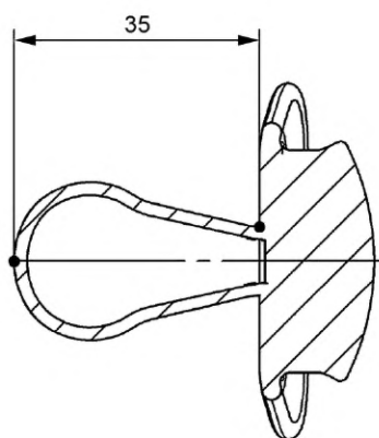
Рисунок 9 — Измерение глубины проникновения баллончика
