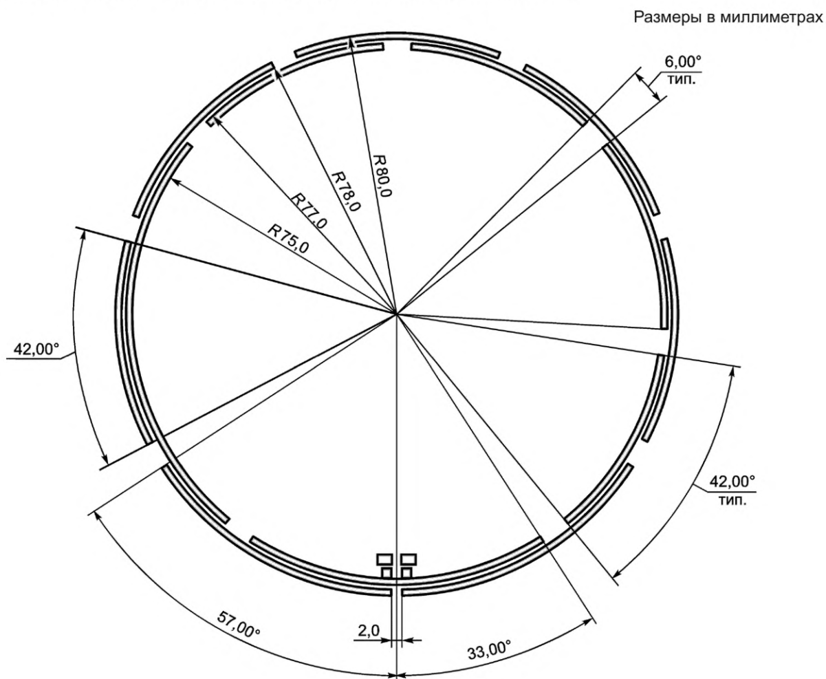
Рисунок С.1 — Конструкция антенны, которая будет использована для измерений индуктивных радиочастотных меток УВЧ
