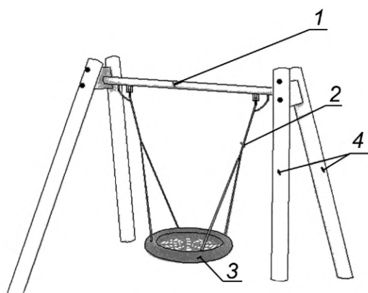
1 — балка; 2 — цепь; 3 — сиденье-гнездо; 4 — стойка
