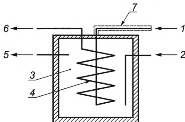
Рисунок А.1 — Испаритель СПГ с водяным или паровым подогревом
