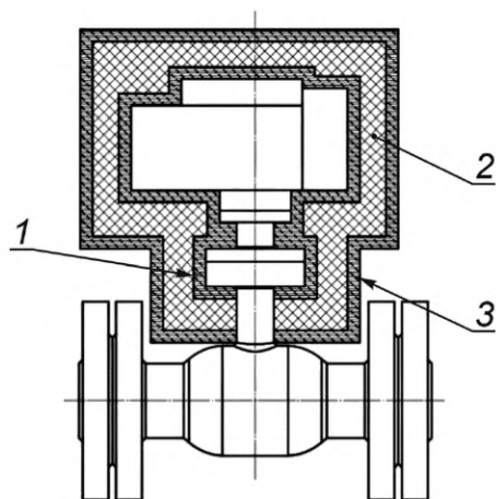
1 — внутренний слой; 2 — теплоизолирующий огнеупорный слой; 3 — внешний слой
