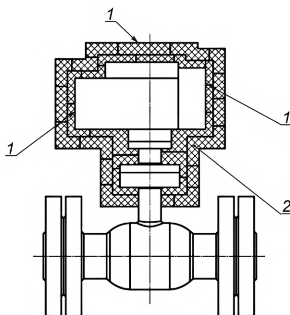
1 — несущие слоисто-ячейки; 2 — огнеупорные теплоизолирующие слоисто-ячейки
