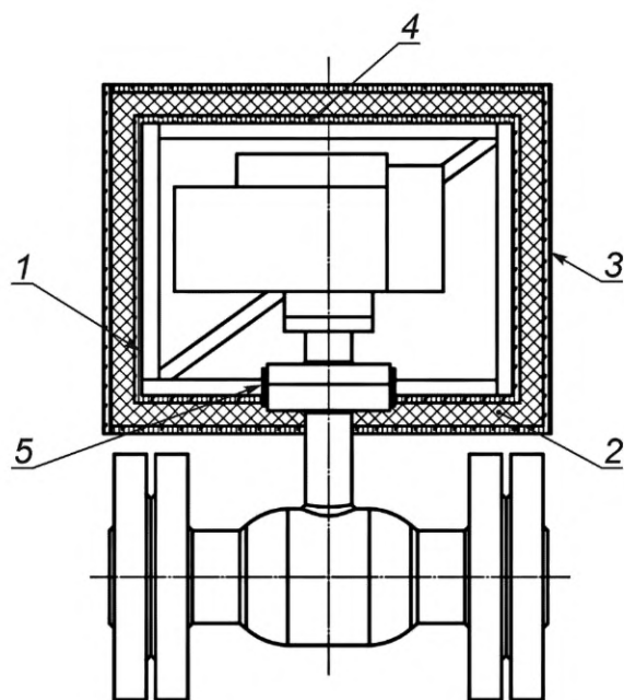
1 — внутренний слой; 2 — теплоизолирующий огнеупорный слой; 3 — внешний слой; 4 — стальной каркас; 5 — хомутовая опора
