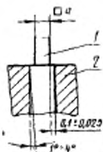
1 — пуансон; 2 — матрица пробивного штампа; а — толщина пуансона
