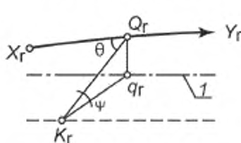
Исходная траектория полета
