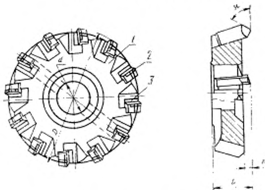
1—корпус; 2—нож (кол. 12); 3—клин (кол. 12)
