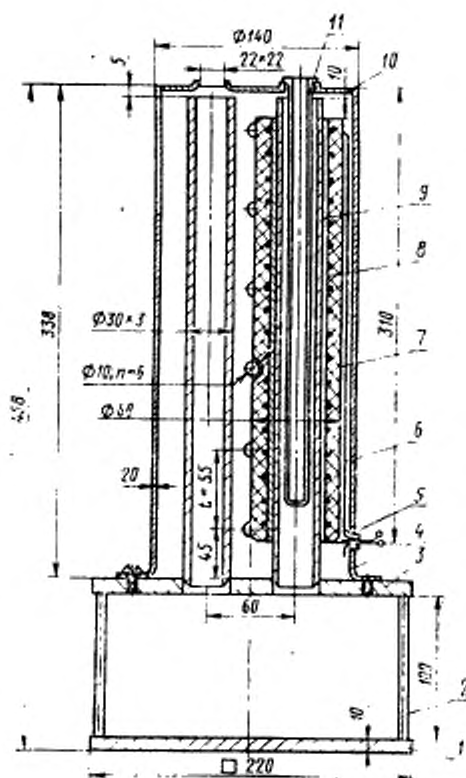
1—опорная плита; 2—опорная стойка; 3—плита; 4—корпус; 5—фарфоровая трубка; 6—провод; 7—изоляция; 8—асбест; 9—труба; 10—крышка; 11—пробирка
