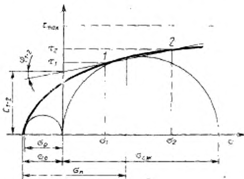
Черт. 4
