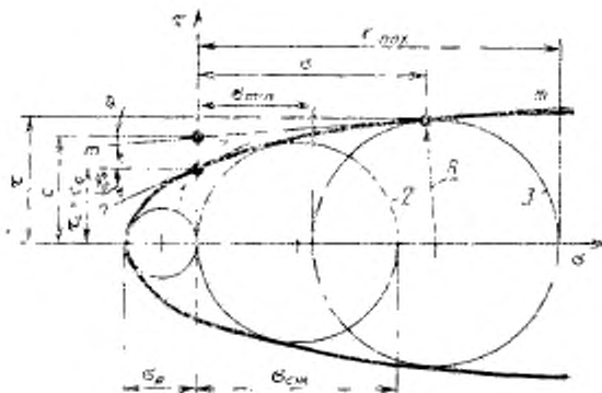
1 — круг одноосного растяжения; 2 — круг одноосного сжатия; 3 — круг объемного сжатия; m — касательная к огибающей в точке ее пересечения с осью \tau ; m_0 — касательная к огибающей в любой точке на ней
