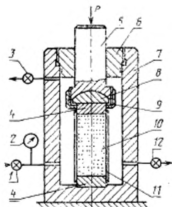
1 — впускной вентиль; 2 — манометр; 3 — вентиль выпуска воздуха; 4 — стальные плиты; 5 — шток; 6 — крышка; 7 — корпус; 8 — сферическая пята; 9 — нажимная гайка; 10 — образец; 11 — изоляция; 12 — выпускной вентиль
