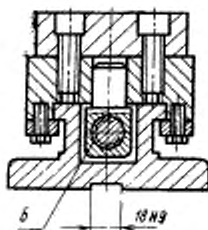
Б-Б поворота
