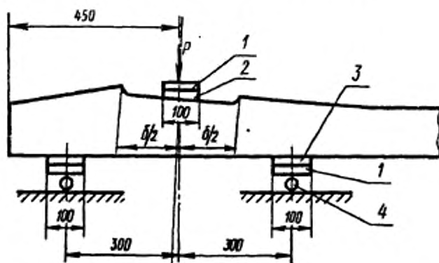
Схема испытания шпалы на трещиностойкость в подрельсовом сечении
