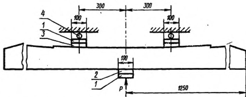
Схема испытания шпалы на трещиностойкость в среднем сечении
