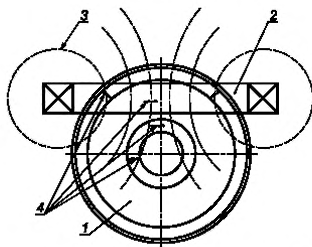
Рисунок В.1 — Схема полюсного намагничивания соленоидом колесного центра
