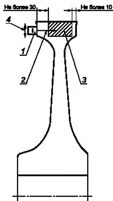
1 — прямой ПЭП; 2 — направление прозвучивания; 3 — зона контроля колесного центра; 4 — направление смещения ПЭП при сканировании
