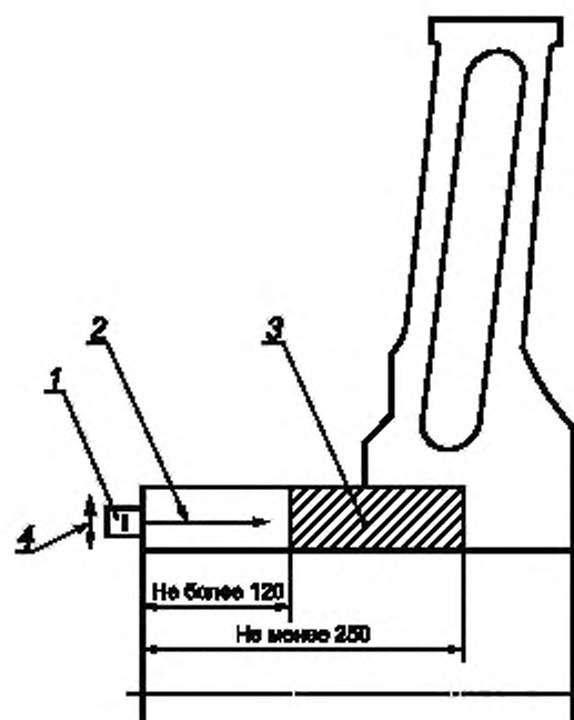
1 — прямой ПЗП; 2 — направление прозвучивания; 3 — зона контроля колесного центра; 4 — направление смещения ПЗП при сканировании
