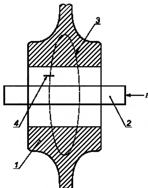
1 — колесный центр; 2 — проводник; 3 — силовые линии магнитного потока, 4 — дефект; I — ток
