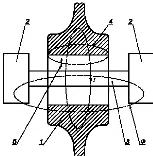
Рисунок В.1 — Схема полюсного намагничивания соленоидом колесного центра
