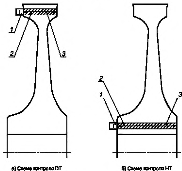
Схемы ультразвукового контроля колесных центров
