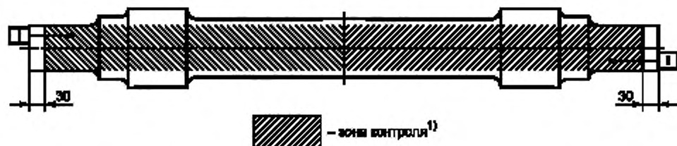
Рисунок 5.2 — Схема А1 и зоны УЗК черновых осей на выявление внутренних дефектов
