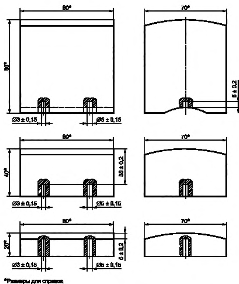
Рисунок А.4 — Меры НК для настройки предельной чувствительности УЗК чистовых полых осей по схеме А2
