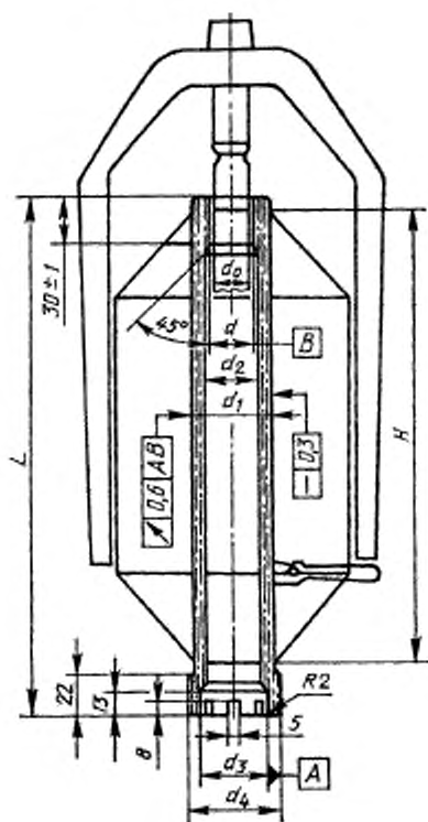
Катушка с выступом
