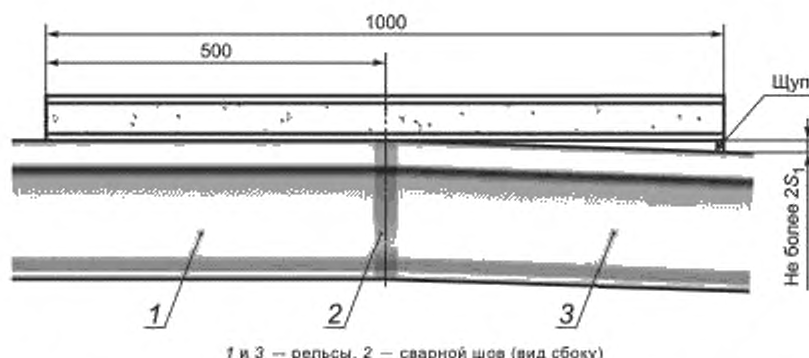
Рисунок 4 — Схема измерения выпуклости стыка РКС по поверхности катания (размеры указаны в миллиметрах)
