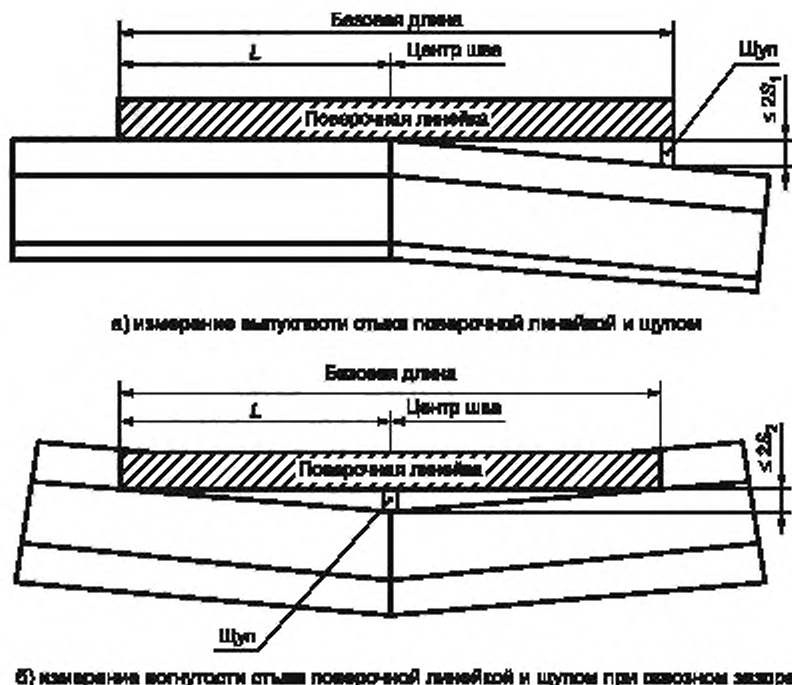
Рисунок 1 — Отклонение рабочих поверхностей стыка РТС от прямолинейности ( L , мм — регламентируемое расстояние между краем поперечной линейки и центром сварного шва)
