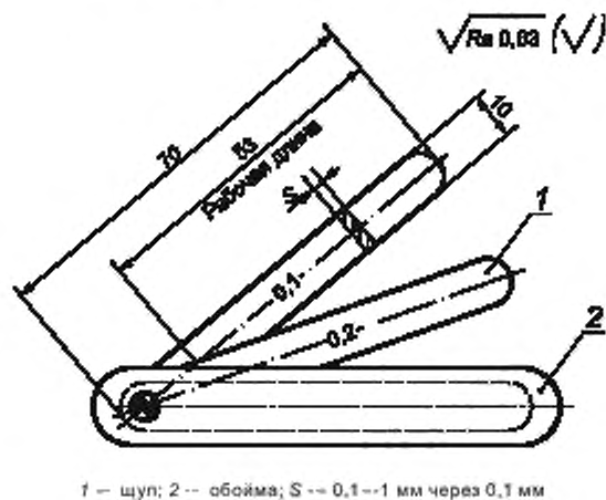
Рисунок Г.1 — Набор плоских щупов
