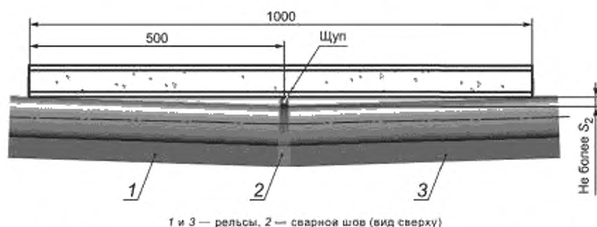
Рисунок 5 — Схема измерения вогнутости стыка РКС по боковой рабочей грани головки рельса (размеры указаны в миллиметрах)
