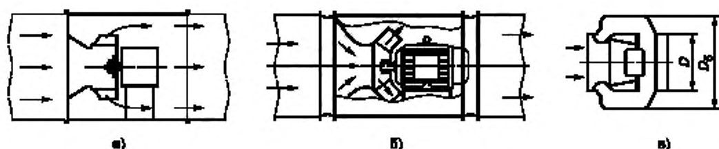
Рисунок 4 — Канальные круглые вентиляторы с цилиндрическим корпусом с радиальным [а)] и диагональным [б)] рабочим колесом, с торообразным корпусом с радиальным рабочим колесом [в)]
