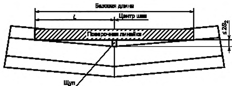
б) измерение вогнутости стыка поверочной линейкой и щупом при сквозном зазоре
