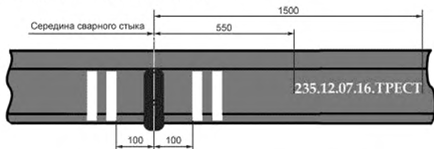
Рисунок 2 — Маркировка РТС (размеры указаны в миллиметрах)
