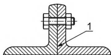
a – плохой вариант (узкая щель, сложно защитить)
