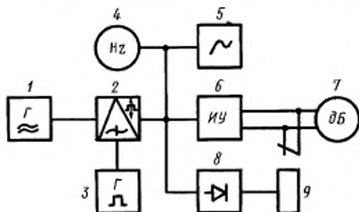
1—звуковой генератор; 2—ключающая схема; 3—генератор прямоугольного напряжения; 4—электронно-счетный частотомер; 5—осциллограф; 6—электрическая часть испытуемого ИУ; 7—показывающий прибор ИУ; 8—мостиковый диодный выпрямитель; 9—реле с временем срабатывания менее 3 мс.
