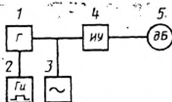
1—генератор сигналов специальной формы; 2—генератор импульсов; 3—осциллограф; 4—электрическая часть испытуемого ИУ; 5—показывающий прибор ИУ
