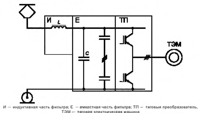
Рисунок А.1 — Принципиальная схема электровоза постоянного тока с однозвенным индуктивно-емкостным фильтром для питания тяговой цепи
