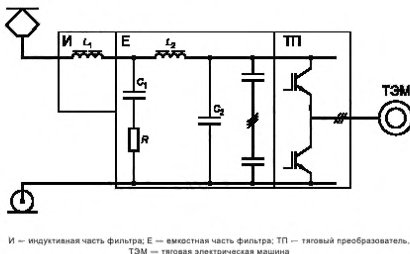
Рисунок А.2 — Принципиальная схема электровоза постоянного тока с двухзвенным индуктивно-емкостным фильтром для питания тяговой цепи
