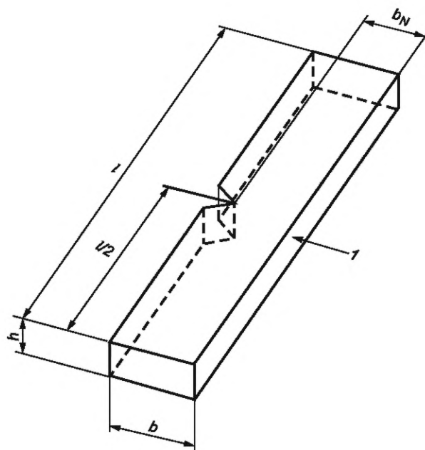
Рисунок 1 — Удар по Шарпи в ребро e образца с надрезом
