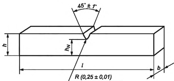
Рисунок 5 — Надрез типа В
