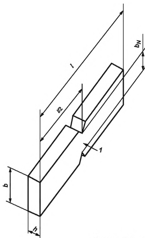
Рисунок В.1 — Образец с двойным V-образным надрезом
