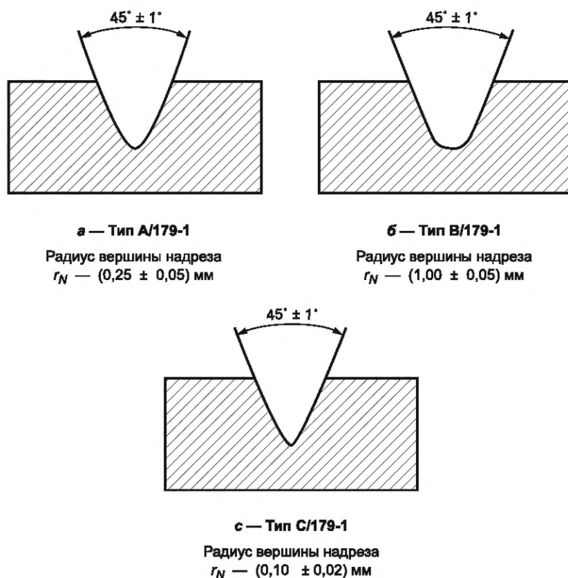
Рисунок 6 — Типы надрезов
