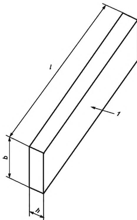
Рисунок 2 — Удар по Шарпи плашмя f
