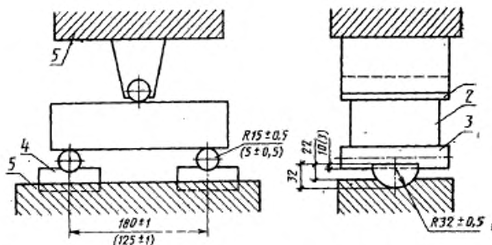
Схема нагружающего устройства
