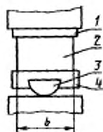
1 — опора для приложения нагрузки (нажимная); 2 — образец для испытания; 3 — дополнительный опорный элемент; 4 — опоры, поддерживающие образец
