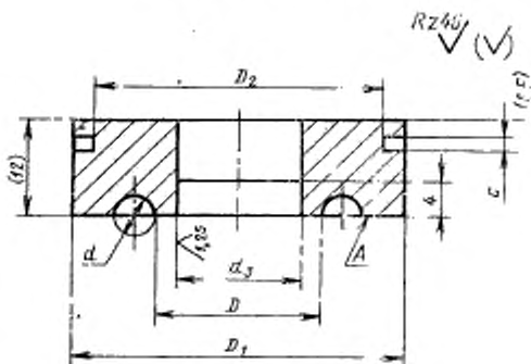
Пуансон (поз. 2)
