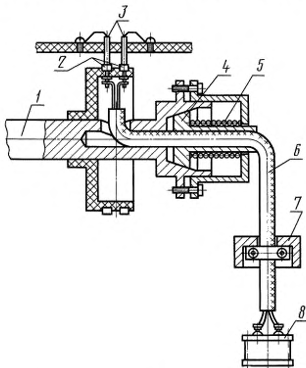
1 — вал; 2 — токосъемные кольца; 3 — щетки; 4 — сегмент; 5 — пружина; 6 — испытуемый шнур; 7 — груз; 8 — конденсатор
