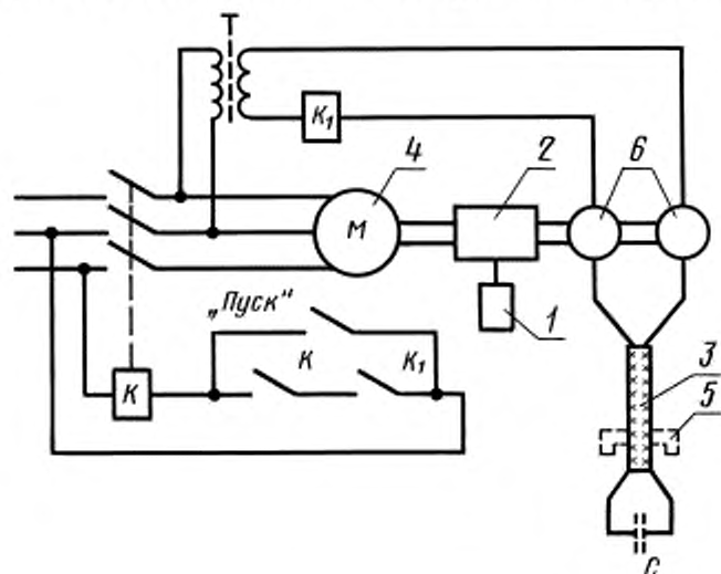
1 — счетчик; 2 — редуктор; 3 — испытуемый шнур; 4 — электродвигатель; 5 — груз; 6 — токоъемные кольца
