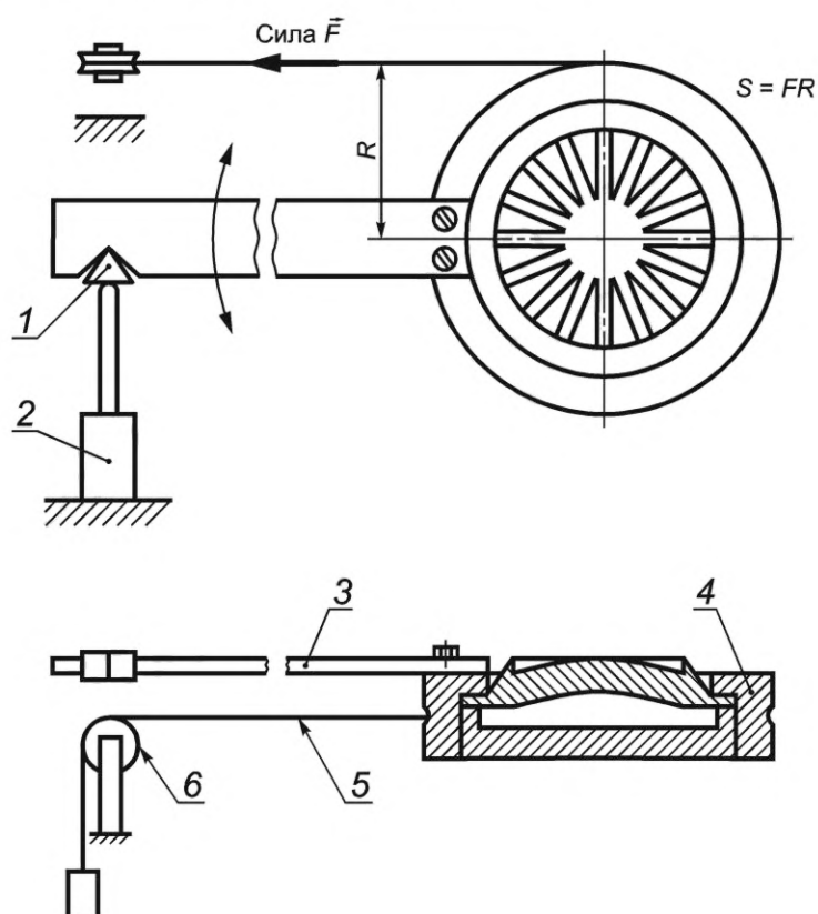
1 — призматическая опора; 2 — датчик перемещения; 3 — плечо рычага; 4 — кольцо; 5 — проволочный трос; 6 — шкив
