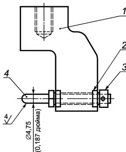
1 — корпус; 2 — два радиальных подшипника; 3 — узкая втулка; 4 — шпиндель из нержавеющей стали типа 300
