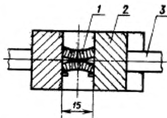
1—образцы; 2—обхваты; 3—стержни.
