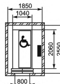
Рисунок А.2 — Пассажирские лифты категории А, рекомендуемые для жилых зданий
