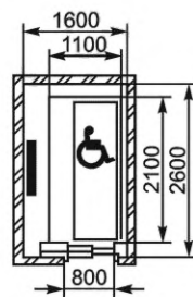
Рисунок А.2 — Пассажирские лифты категории А, рекомендуемые для жилых зданий
