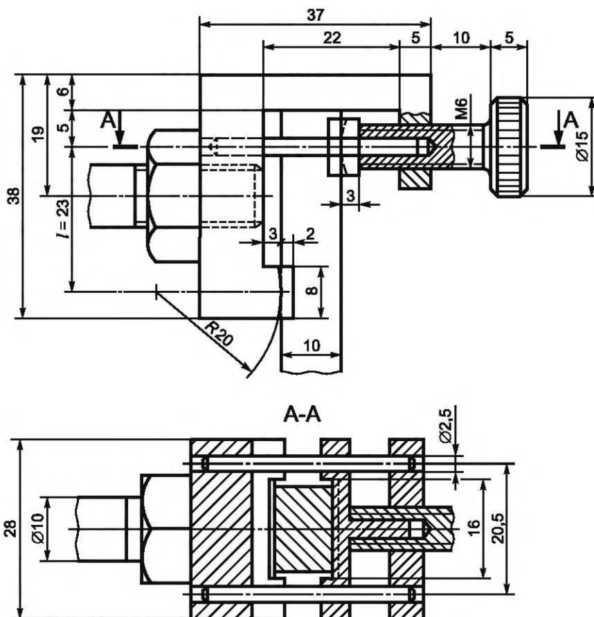
Рисунок 3 — Верхняя зажимная головка для образца 1
