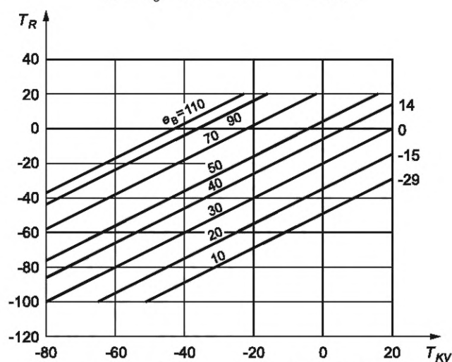
T_R — расчетная эталонная температура; T_{KV} — температура испытания материала на удар; e_B — эталонная толщина Рисунок Г.5 — Расчетная эталонная температура и температура испытания на удар, условия термообработки после сварки PWHT, для R_e \leq 460 МПа и KV \geq 40 Дж
