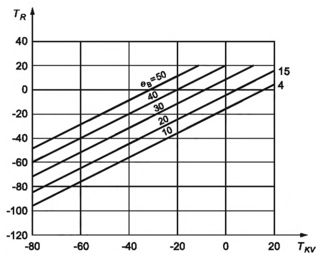
Рисунок Г.11 — Расчетная эталонная температура и температура испытания на удар аустенитно-ферритных сталей в состоянии после сварки АW, для R_e \leq 550 МПа и KV \geq 40 Дж
