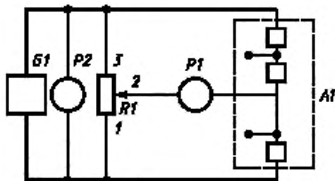
GI — источник напряжения постоянного тока; RI — проверяемый резистор; P1, P2 — вольтметр постоянного тока; AI — образцовый делитель напряжения или другое устройство, формирующее образцовую функциональную характеристику
