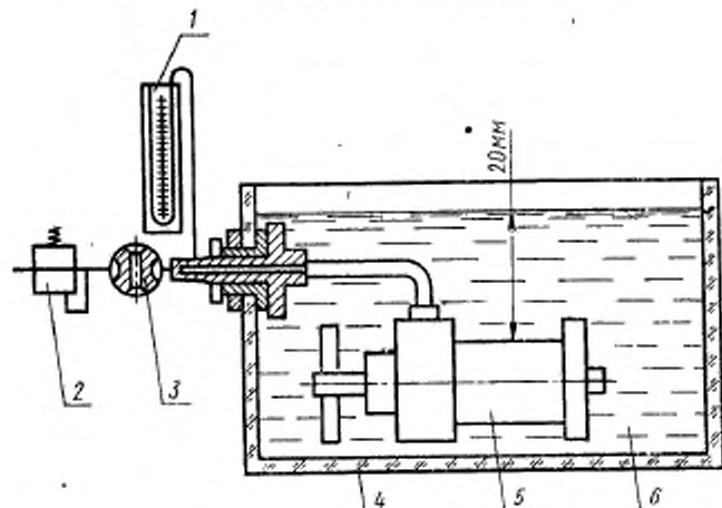
1—манометр по ГОСТ 9933—75; 2—регулятор давления; 3—кран; 4—ванна; 5—испытываемый фильтр; 6—бензин В-70.
