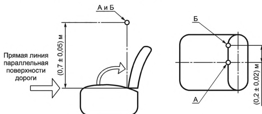
Рисунок 1 — Место записывающего микрофона относительно сиденья
