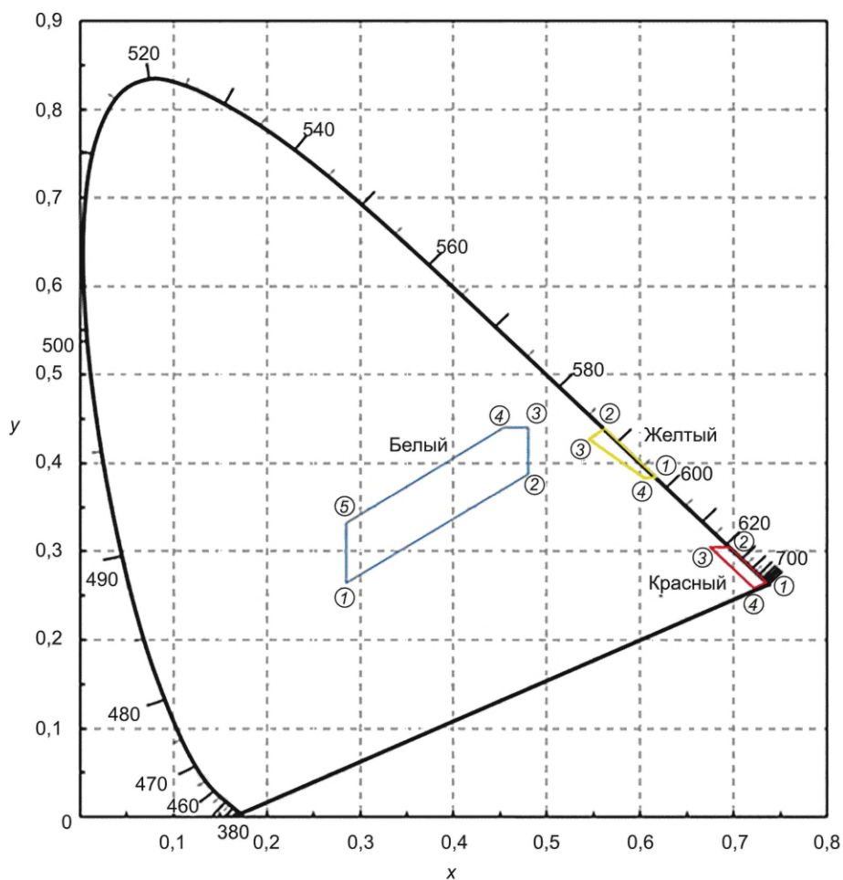
Рисунок А.1 — График координат цветности x , y с областями цветностей излучения белого, красного и желтого цветов».
