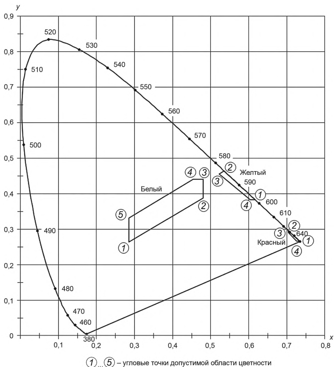
Рисунок А.1 — График координат цветности x , y с областями цветности излучения белого, красного и желтого цвета
