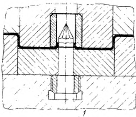
1 — проколочный пуансон по ГОСТ 24533—80
