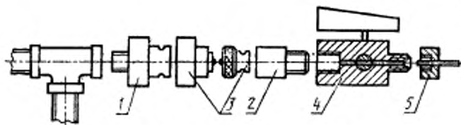
1 — запорный клапан, постоянно подсоединенная часть быстроразъемного соединения; 2 — съемная часть быстроразъемного соединения (если применяется); 3 — защитные крышки; 4 — сферический край; 5 — насадок
