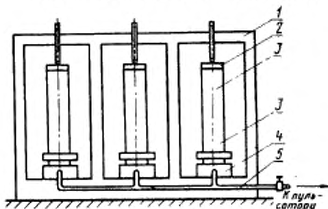
1—рама машины; 2—вертикальные винтовые стойки с оголовниками; 3—образцы; 4—гидрозомкрат; 5—маслопровод.
