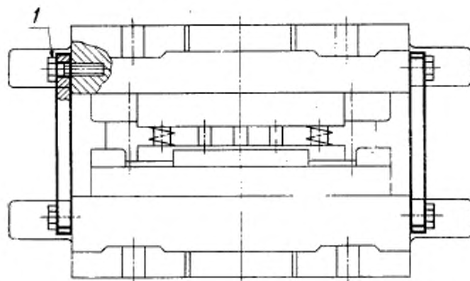
1—болт по ГОСТ 7805—70
