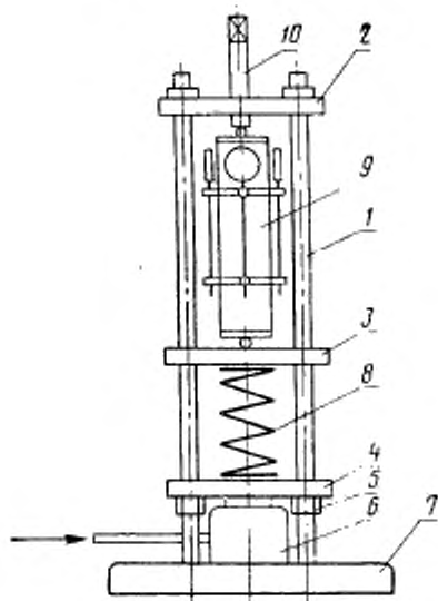
1—стойки; 2—верхняя траверса; 3—средняя траверса; 4—нижняя траверса; 5—гайки; 6—гидравлический домкрат; 7—образец; 8—спиральная пружина; 9—бетонный образец; 10—установочный винт.
