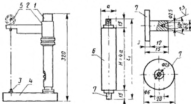
1—стойка; 2—кронштейн; 3—конусообразный выступ; 4—нижняя опора; 5—индикатор; 6—образец; 7—репер; a —размер стороны поперечного сечения образца; H —высота образца; L_{изм} —база измерений.
