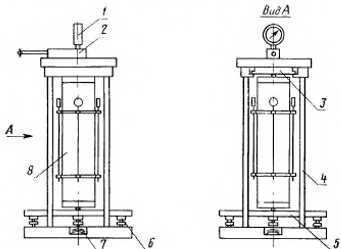
1—образцовый манометр; 2—гидравлический домкрат плунжерного типа с гибкой диафрагмой; 3—поршень домкрата; 4—стойки; 5—опорная плита; 6—регулирующие винты; 7—тарельчатые пружины; 8—образец.
