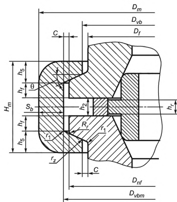
Рисунок 4 — Бугельное соединение
