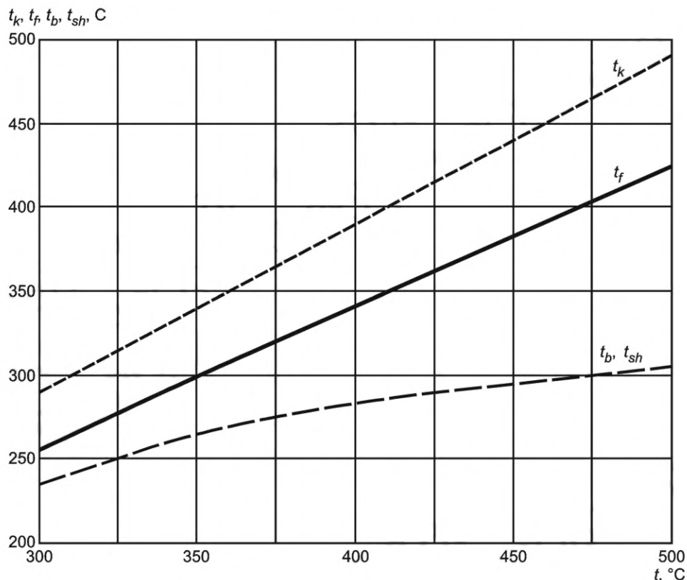
Рисунок 3 — Зависимость температуры деталей уплотнения ( t_{f1} , t_{f2} , t_k , t_b , t_{sh} , ^\circ\text{C} ) от температуры внутренней среды ( t , ^\circ\text{C} )
