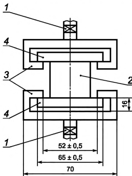
1 — карданный шарнир; 2 — образец; 3 — захват; 4 — колодки
