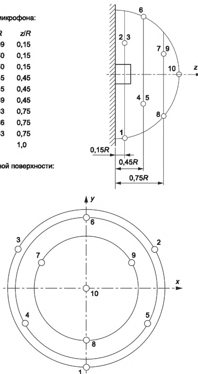
Рисунок 101 — Полусферическая измерительная поверхность с 10 позициями микрофона для вентиляторов, встраиваемых в отверстие стены или окна, и настольных вентиляторов, устанавливаемых на стене
