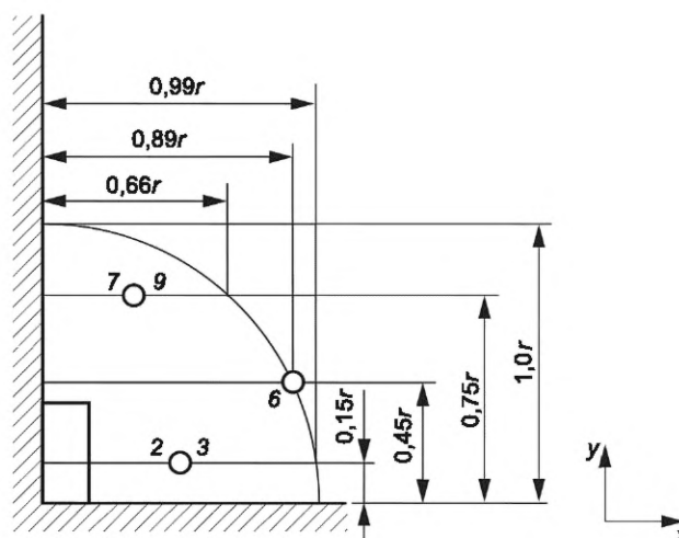
Рисунок 5 — Измерительная поверхность и точки измерений для небольших пристенных напольных изделий
