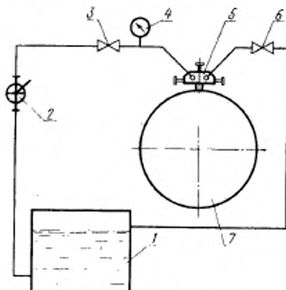
1—емкость; 2—магнитный насос; 3, 6—вентили; 4—манометр; 5—головка; 7—разделитель.
