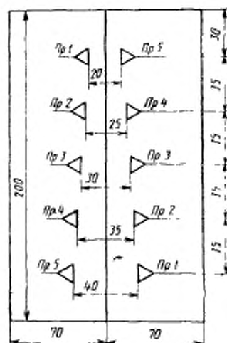
Огнеупорная подставка с пироскопами
