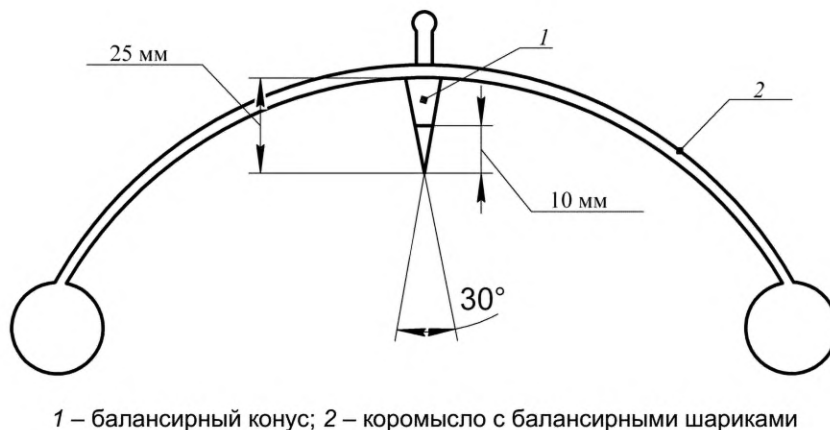
Рисунок 3 – Балансирный конус
