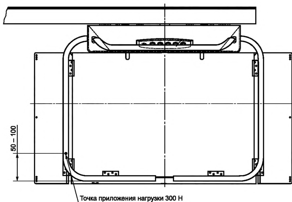
Рисунок Б.3 — Точка приложения нагрузки 300 Н
