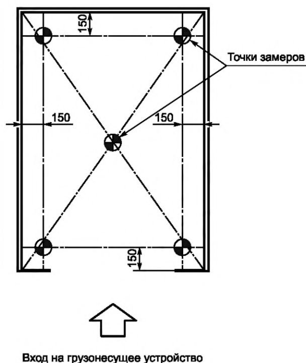
Рисунок Б.2 — Схема расположения контрольных точек
