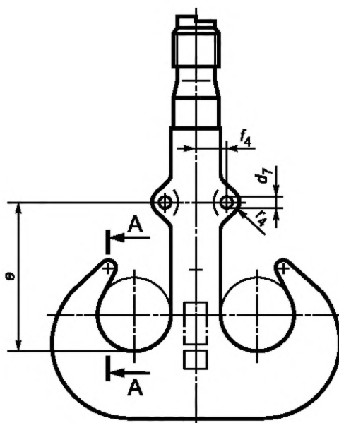
Рисунок 9 — Размеры для двурогих крюков категории IV
