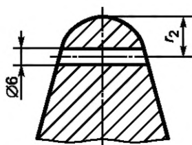
Рисунок 7 — Размеры для штампованных однорогих крюков категории I из заготовок исполнения IV от № 10 до № 40 включительно
