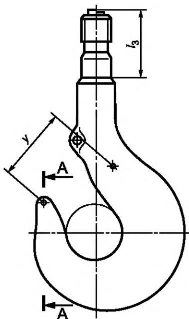
Рисунок 7 — Размеры для штампованных однорогих крюков категории I из заготовок исполнения IV от № 10 до № 40 включительно
